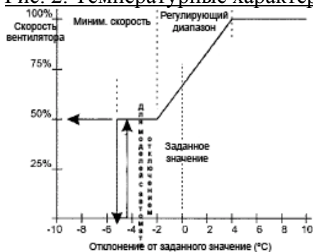
Рис. 2. Температурные характеристики
